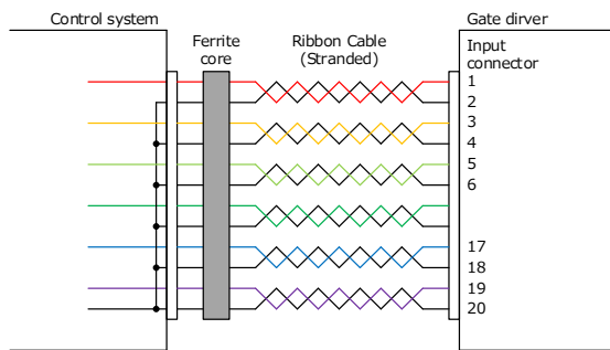
Input cables
